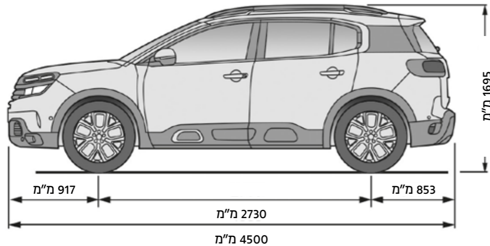
מידות במ"מ
